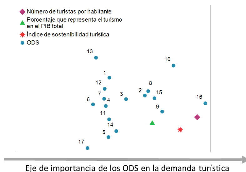
Gráfica 4. Representación del tercer eje del análisis factorial que muestra el grado de implicación de los distintos ODS con la demanda turística del país.
